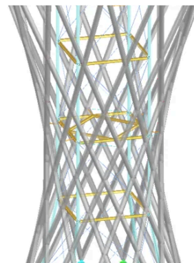
Das Statikmodell der Doppelhelix mit Montageturm und Richtstreben. (c) PORR
