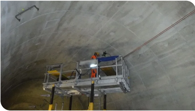
Die Verankerungsdübel für die Deckenstromschienen wurden von einer gleisgebunden Arbeitsbühne aus eingeklebt. Quelle: CPC/Chladek
