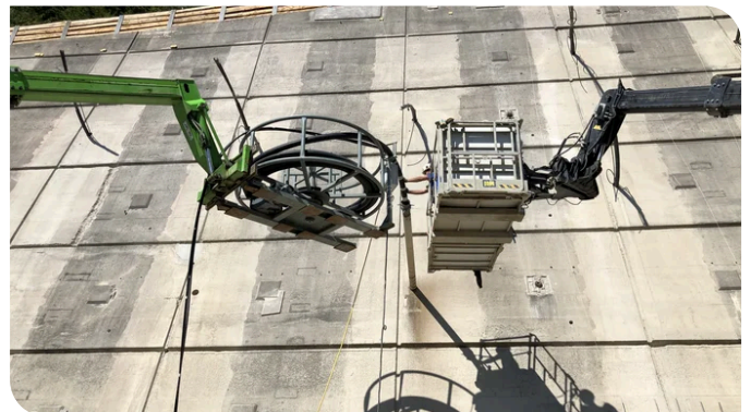
In der Ankerwand Hochmais wurden insgesamt 167 Litzendaueranker mit einer Gesamtankerlänge von 4.615 m verbaut. Quelle: PORR Spezialtiefbau
