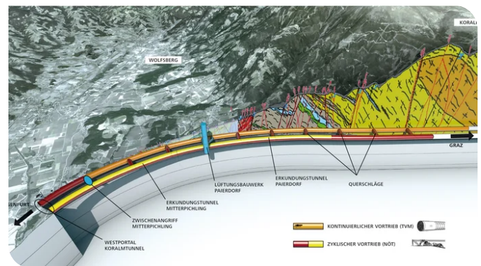
Übersicht Koralmtunnel KAT3. Die Darstellung zeigt die Nord- und Südröhre mit deren Verbindungen mit den Querschlägen. Quelle: ÖBB
