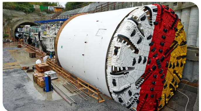
Die Montage der TVM "KORA" wurde in der Baugrube Mitterpichling durchgeführt. Der Bohrkopf ist in den Kärntner Landesfarben gehalten. Quelle: Toni Rappersberger
