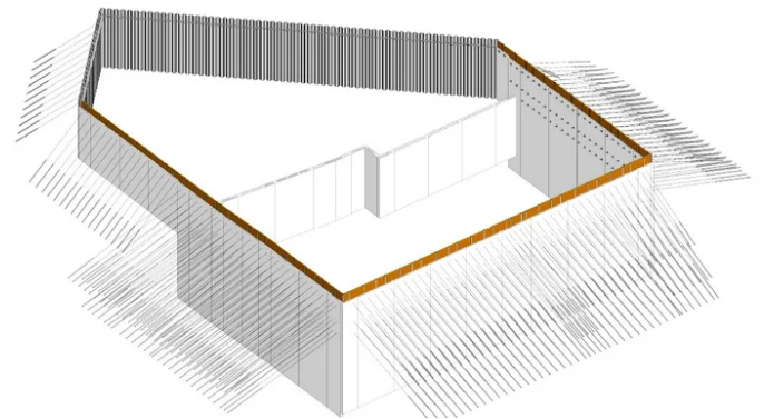
Darstellung der Baugrube als 3D Modell. Bild: isg
