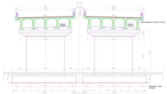
Brückenquerschnitt der größten Fertigteilträger mit einer Länge von 40,75 m und einer Höhe von 2,10 m. Bild: PORR AG
